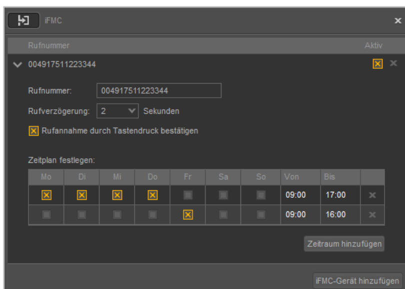
Abbildung 38 - Beispiel für eine iFMC-Konfiguration
