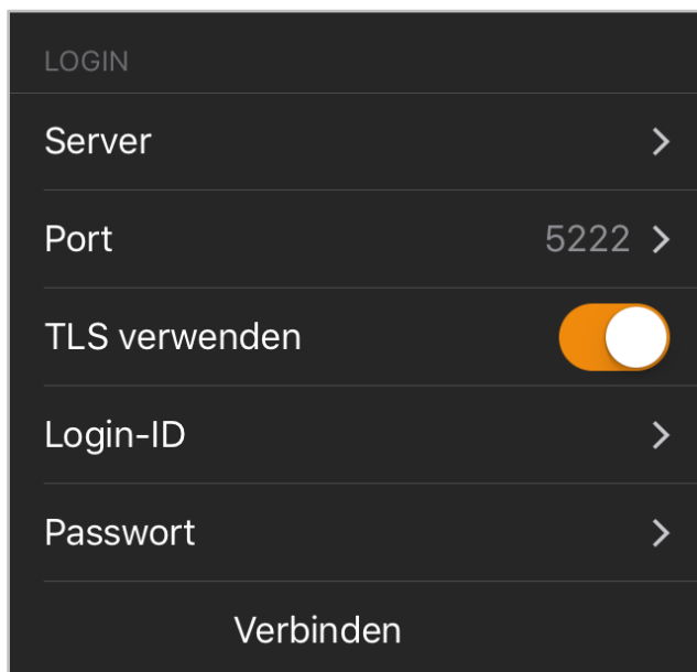
Abbildung 1 – Login-Screen
