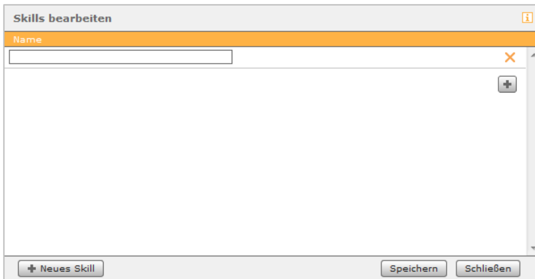
Abbildung 18 - -kills hinzufügen
