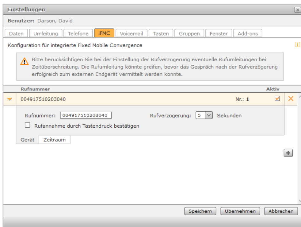
Abbildung 35 - Beispiel für eine iFMC Konfiguration
