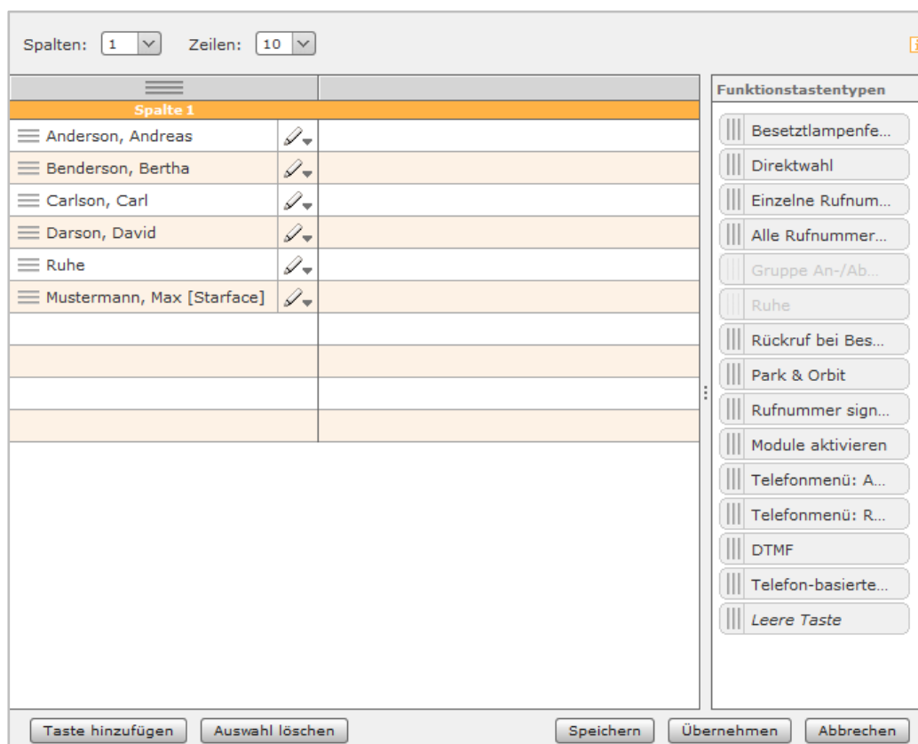
Abbildung 22 - Anlegen einer Funktionstaste per Drag&Drop
