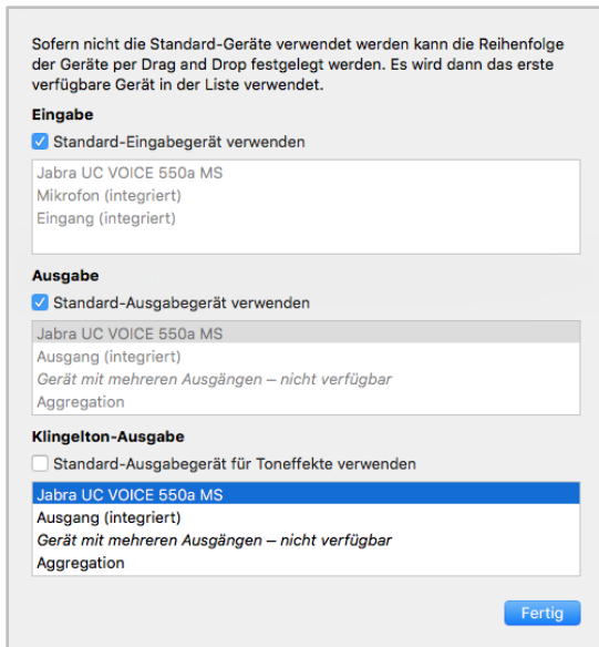
Abbildung 14 - Audioeinstellungen
