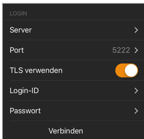
Abbildung 15 – Login-Einstellungen
