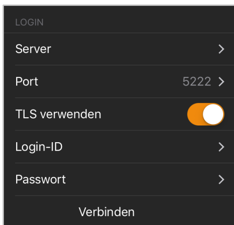
Abbildung 15 – Login-Einstellungen
